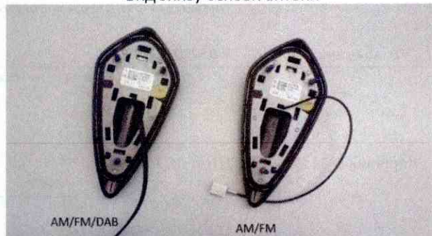
Вид знизу основи антени
